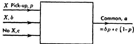
FIG. 15. Selector.
