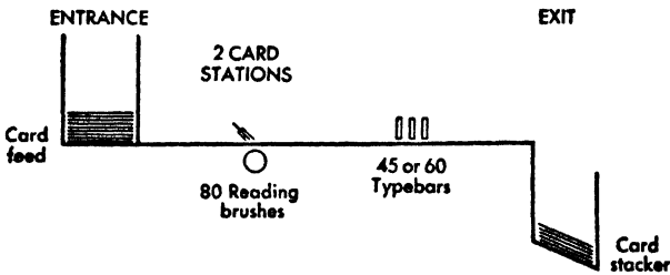
FIG. 8. Interpreter.
