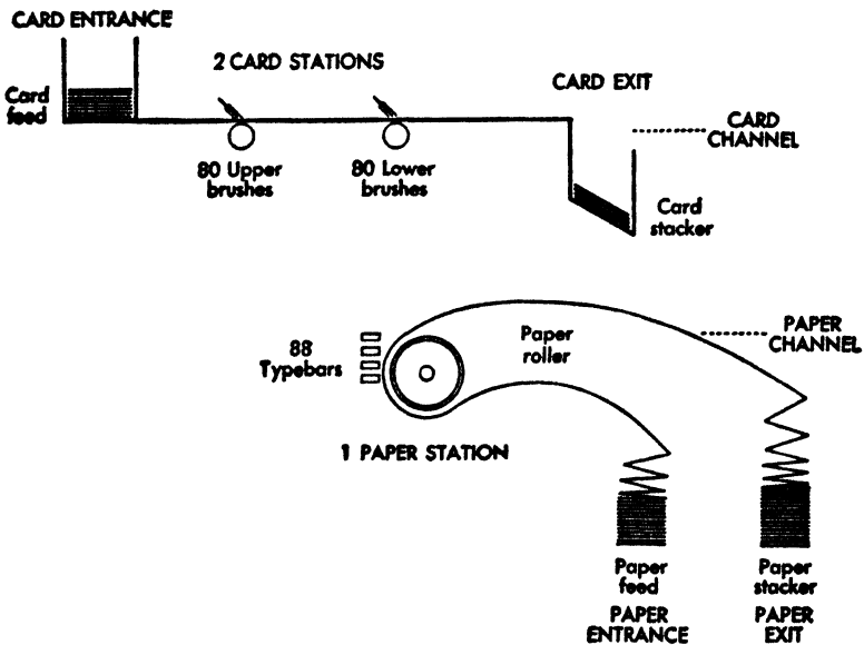
FIG. 12. Tabulator.
