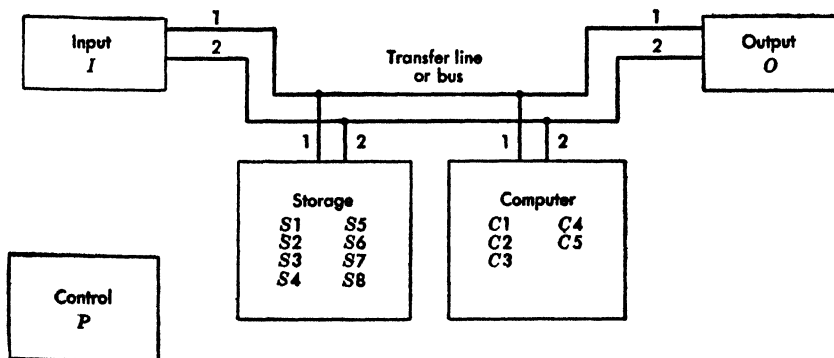
FIG. 4. Scheme of Simon.
