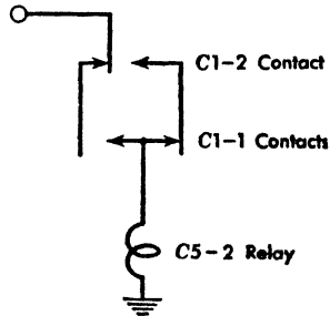
FIG. 7. Negation—left-hand digit.
