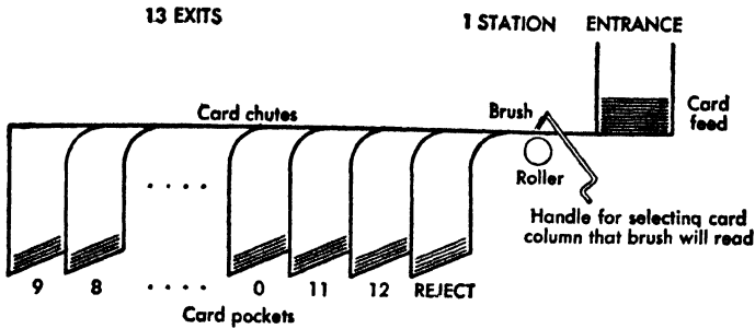
FIG. 7. Sorter.
