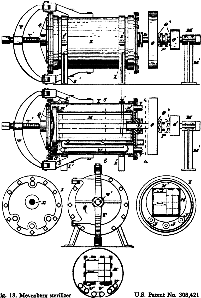
Fig. 13. Meyenberg sterilizer
