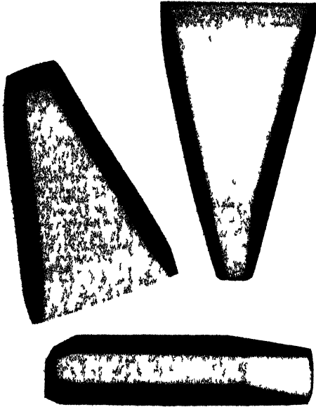
Fig 4. Lactose crystals
