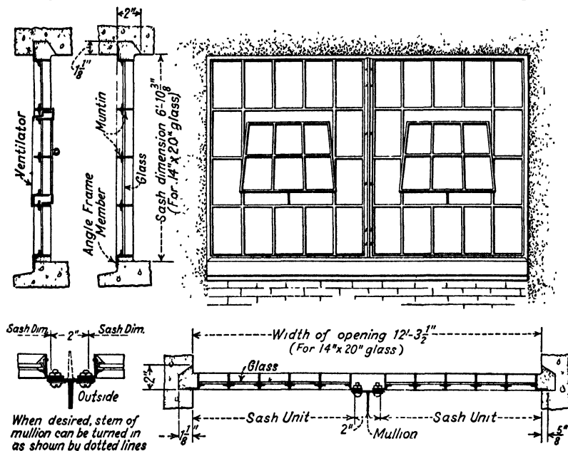
FIG. 235.—Window Sash. (See p. 700.)
