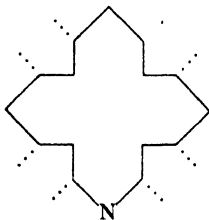
Fig. 21. Monoazaporphyrins.
