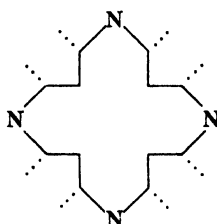
Fig. 23. Tetraazaporphyrins.
