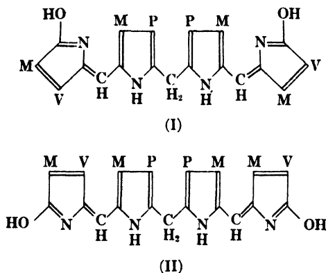
Fig. 8. Linear formulas of bilirubin.
