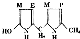
Fig. 4. Bilirubinic acid.
