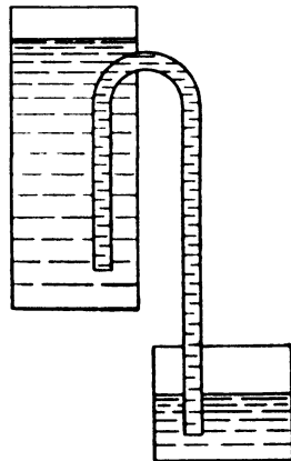
FIG. 56. Automatic Siphon.
