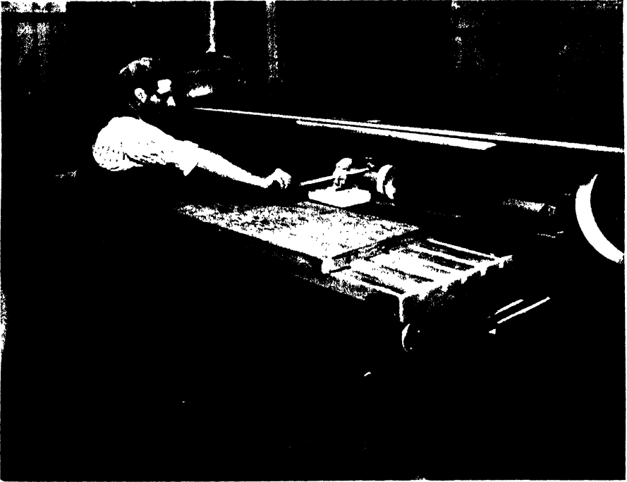
FIG. 60.—BELT SANDER.
