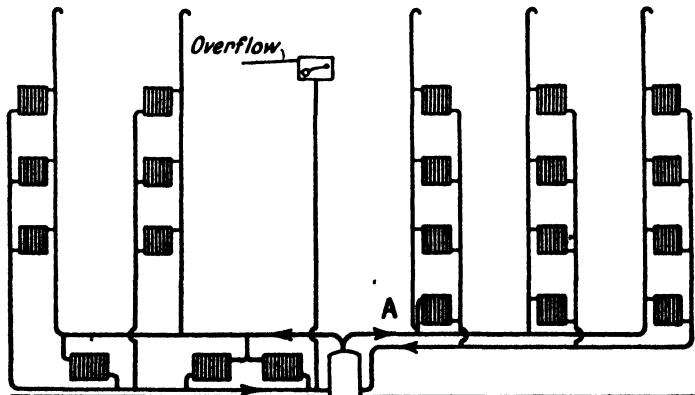
Fig. 11. — TWO-PIPE UP-FEED SYSTEM.—1
