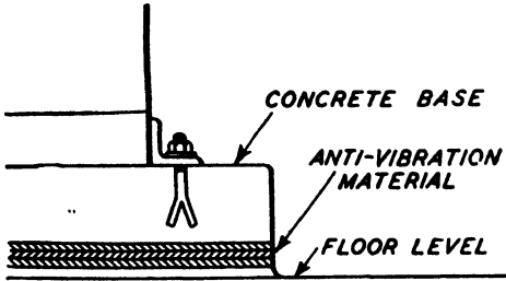
Fig. 8.—METHOD OF INSULATING CENTRIFUGAL FAN
