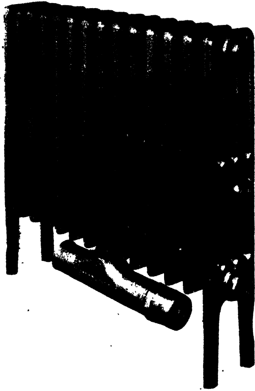
Fig. 9.—ELECTRO-VAPOUR RADIATOR
