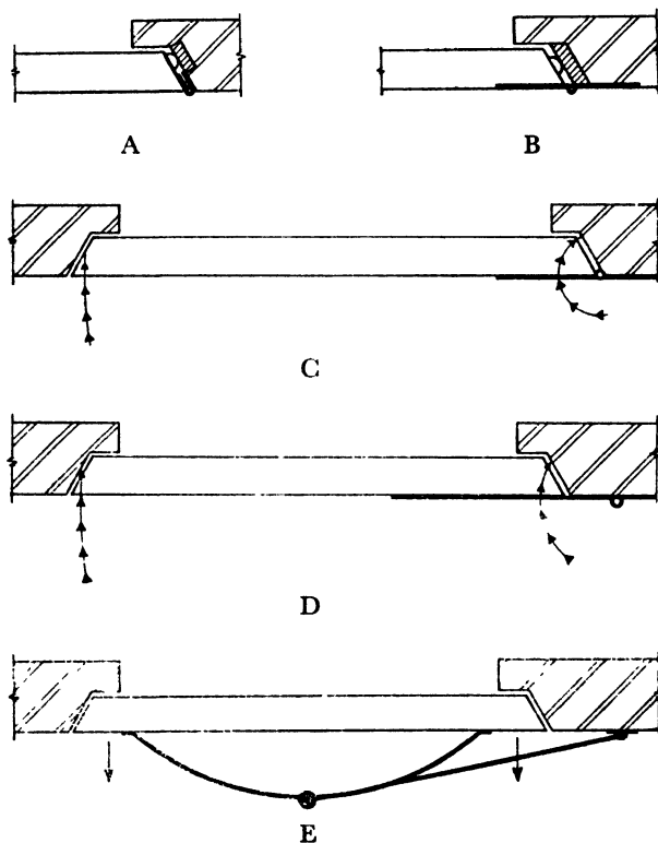
FIG. 40 HINGES
