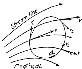
FIG. 21.—Line integral.
