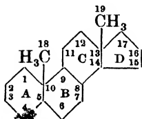
Androstane.
