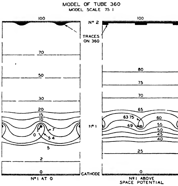
Fig. 4—Equipotential maps on scale model.
