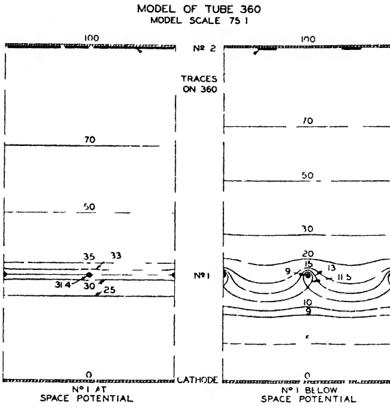
Fig. 3 Equipotential maps on scale model
