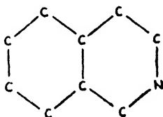
“ Iso-quinoline ” skeleton
