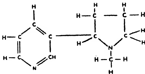
Nicotine
