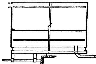
FIG. 15.—Lime Slacker.
