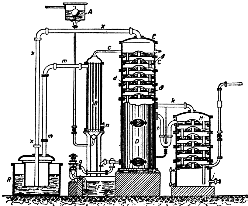
FIG. 1.—Feldmann's Ammonia Still.
