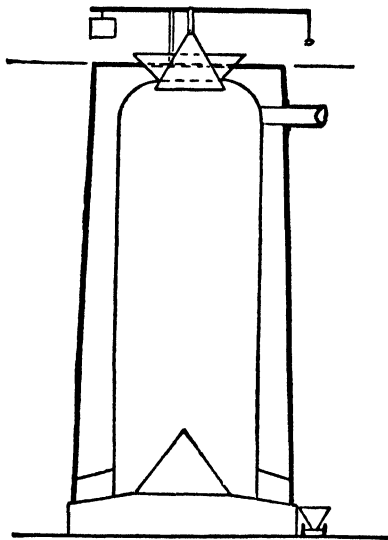
FIG. 14.—Lime-Kiln.
