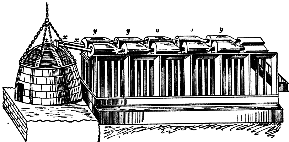
FIG. 2.—Iodine Still.
