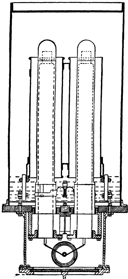
FIG. 9.—Gérard System.
