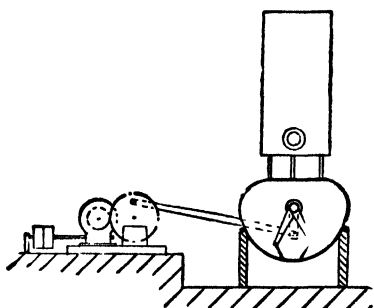
FIG. 16.—Thelen Pan.
