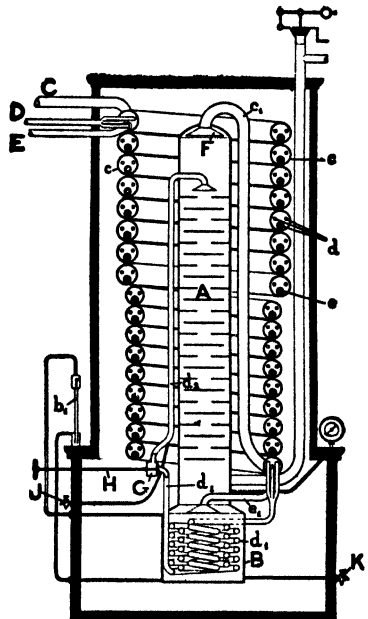
FIG. 14.—Linde Separator.
