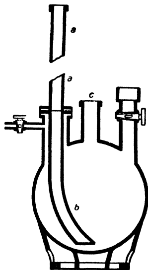
FIG. 4.—Acid "Egg."
