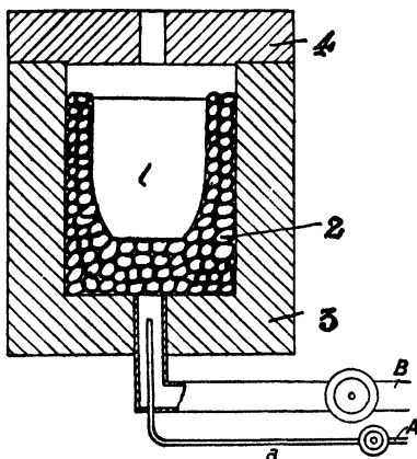
FIG. 3.—Utilisation of Liquid Fuel.
