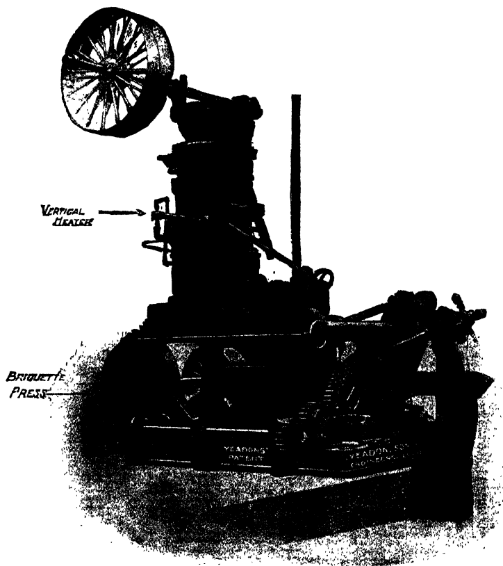
FIG. 1.—Yeadons' Briquette Machine.
