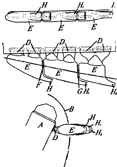
FIG. 325. Rolls Royce ejector type silencer.
