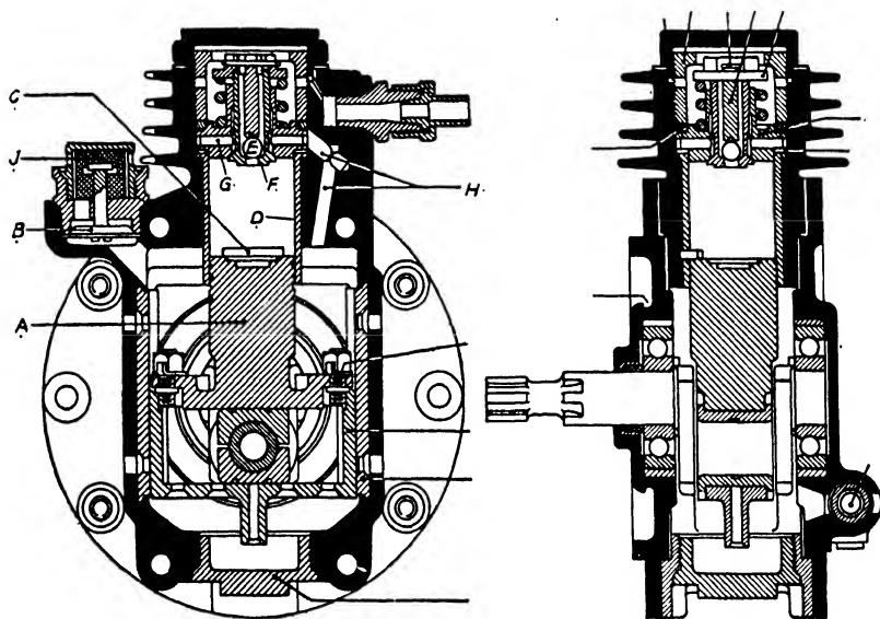
FIG. 349. The B.T.H. air compressor.
