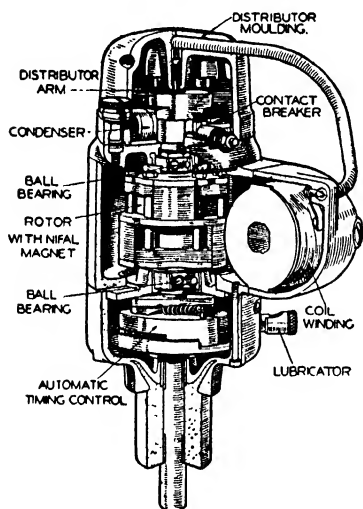
FIG. 288. Automobile type of camshaft speed magneto. (Lucas).
