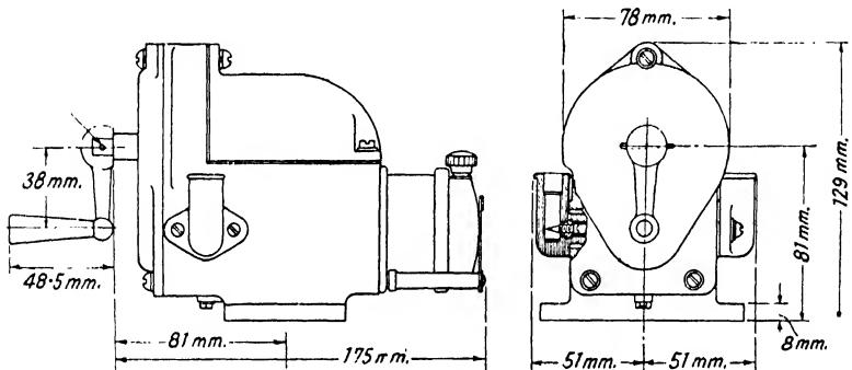
FIG. 332. B.T.H. hand starting magneto.
