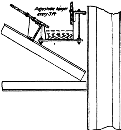
Fig. 142.—Valley gutter
