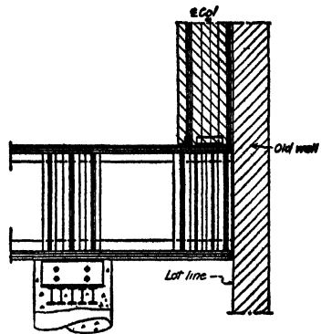
FIG. 56.—Cantilever girder.
