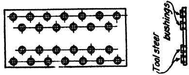
FIG. 33.—Reaming templet.
