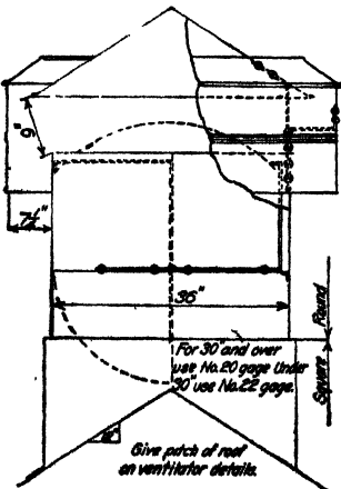
FIG. 138.—Circular ventilator.
