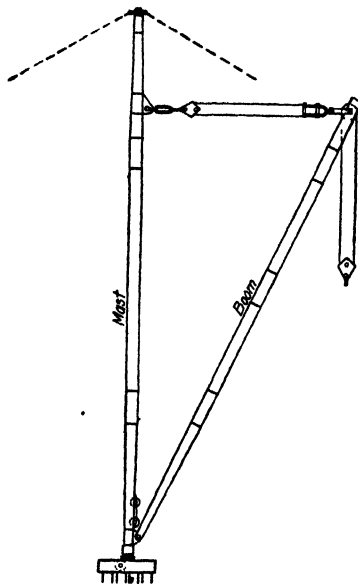
FIG. 7.—Twelve-ton guy derrick.
