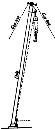
FIG. 10.—Gin pole.
