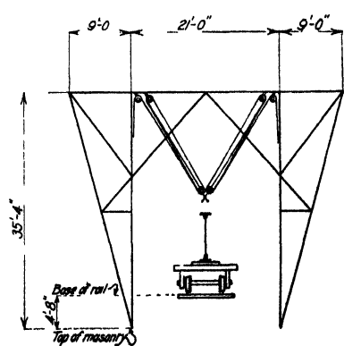
FIG. 3.—Gallows frame.
