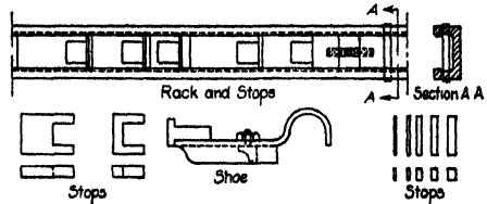
FIG. 6.—Hunter bar.
