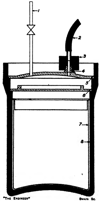
FIG. 8.—BARCO ANNEALING POT.
