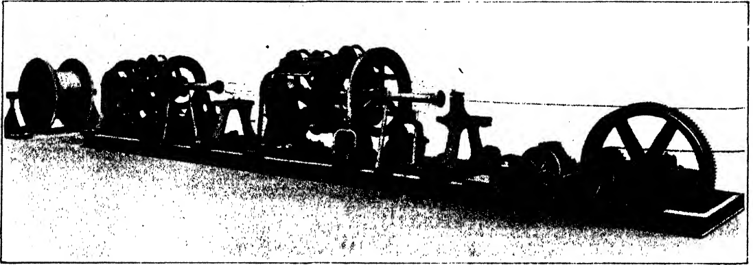
FIG. 113.—DOUBLE-TANDEM STRANDER.
