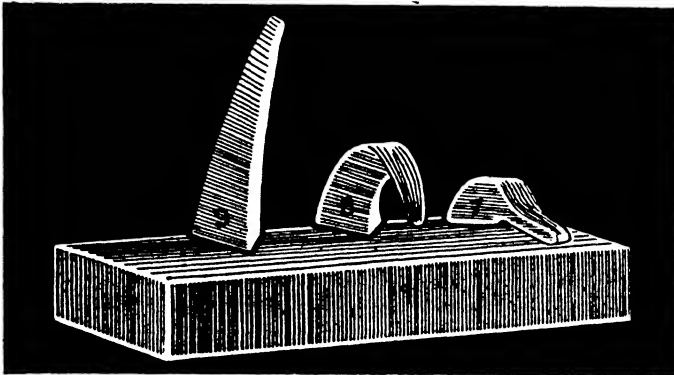
FIG. 56.—Séger Cones.
