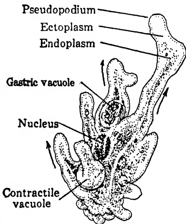
FIG. 13. — Amoeba proteus .
