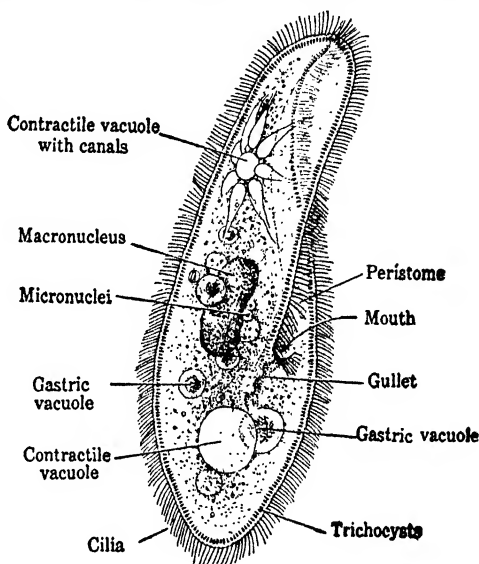
FIG. 27. — Paramecium aurelia .
