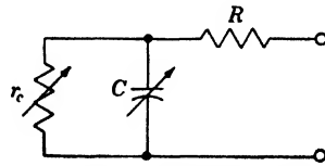
FIG. 11-21.—Equivalent circuit of a crystal rectifier.
