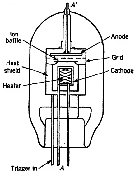
FIG. 10-41.—Hydrogen thyatron.
