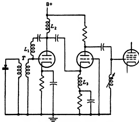
FIG. 12-5.—Triode input circuit.
