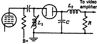
FIG. 12-9.—Diode detector.
