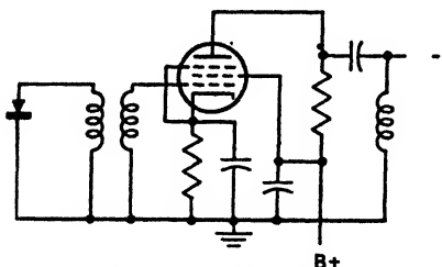
FIG. 12-4.—Pentode input circuit.
