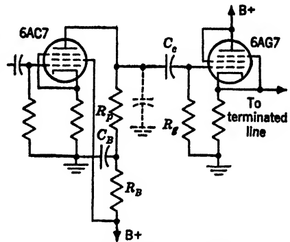
FIG. 12-10.—Video amplifier.
