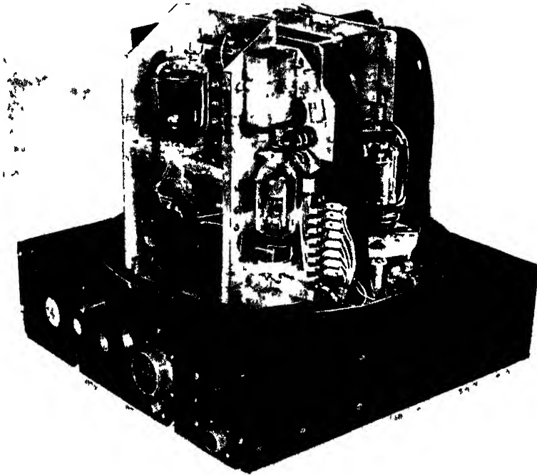
FIG. 10 35.—Hard-tube airborne pulser.
