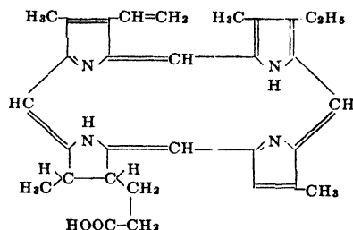
Porphochlorin
