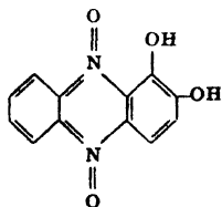
Lyochromes 199
