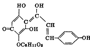
Carthamin
