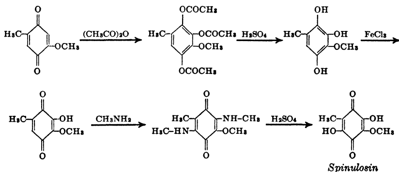
Spinulosin
