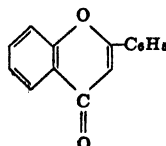
Flavone
