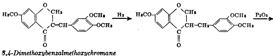
3,4-Dimethoxybenzalmethoxychromane
