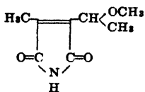
Imide (m.p. 64°)
