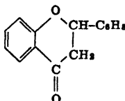
Flavanone
