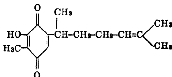
Perezone
