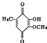
Fumigatin
