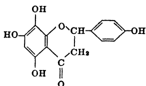
Carthamidin
