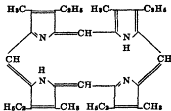
Aetioporphyrin I
