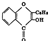
Flavonol (enol form)
