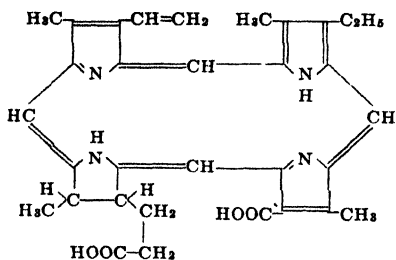
Rhodochlorin
