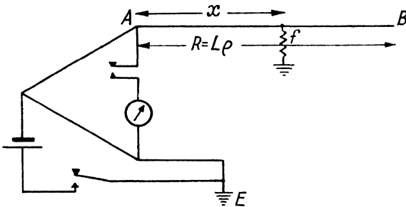
FIG. 124. BLAVIER TEST
