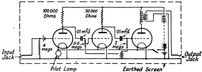
FIG. 130. J. H. SAVAGE'S AMPLIFIER UNIT
