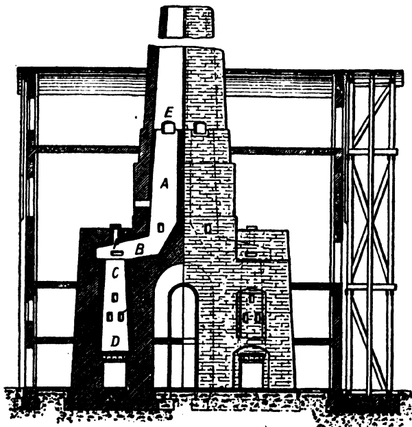
FIG. 11.—Dietzsch Kiln.
