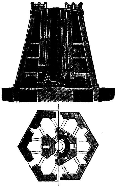
FIG. 3.—Rüdersdorf Kiln.
