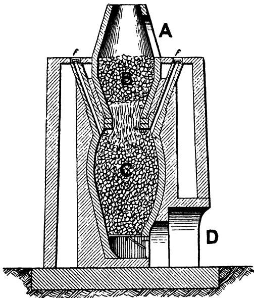
FIG. 2.— The Aalborg Lime Kiln.
