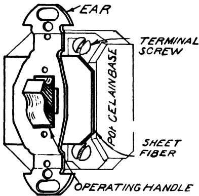
Fig. 10. Tumbler Switch
