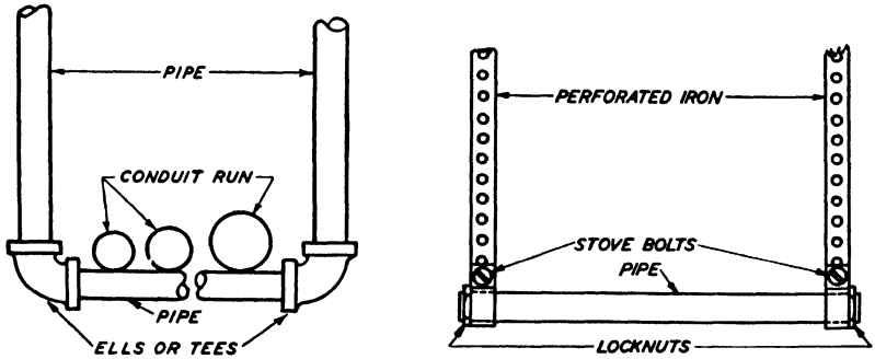
Fig. 40. A Trapeze Conduit Hanger
