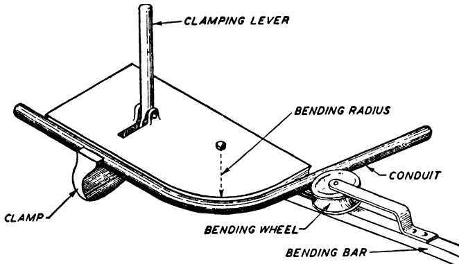
Fig. 25. Bench Type Conduit Bender for 1/2- and 3/4- Inch Conduit
