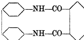
IV. Phthalyl-benzidine 4
