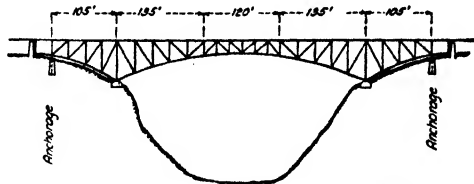
FIG. 30.—Arroya Del Chico Bridge, Mexico.
