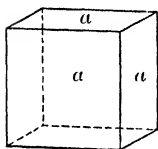
Fig. 11. Cube.
