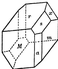
Fig. 186. Axinite.
