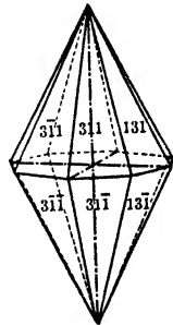
Fig. 84. Ditetragonal Pyramid.
