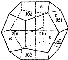
Fig. 52. Pyritohedron.
