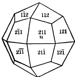
Fig. 40. Trapezohedron.
