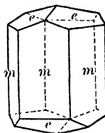
Fig. 127. Calcite.
