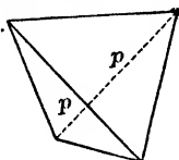
Fig. 98. Sphenoid.
