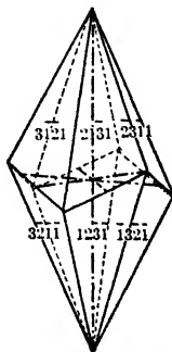
Fig. 132. Scalenohedron.
