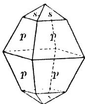
Fig. 151. Sulphur.
