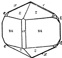
Fig. 157. Brookite.
