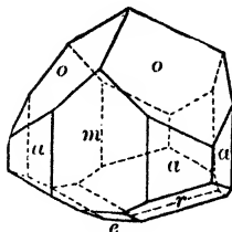
Fig. 139. Tourmaline.
