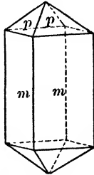
Fig. 86. Zircon.
