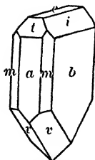
Fig. 162. Calamine.
