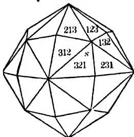
Fig. 46. Hexoctahedron.
