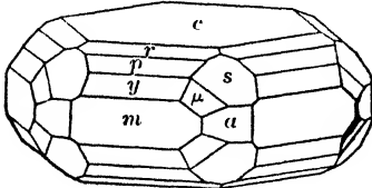
Fig. 115. Apatite.
