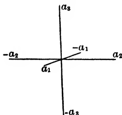
Fig. 23. Isometric Axes.
