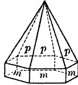
Fig. 116. Zincite.
