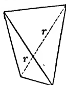
Fig. 97. Sphenoid.
