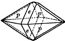
Fig. 89. Vesuvianite.
