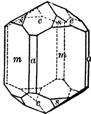
Fig. 91. Rutile.
