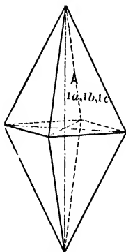
Fig. 7. Orthorhombic Pyramid.
