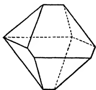
Fig. 18. Distorted Octahedron.
