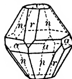
Fig. 130. Corundum.
