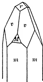
Fig. 135. Calcite.
