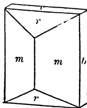
Fig. 153. Staurolite.
