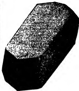
Fig. 293. Manebach Twin.
