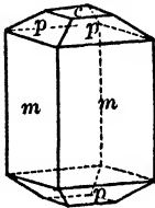
Fig. 89. Vesuvianite.
