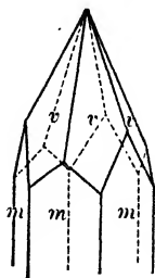
Fig. 134. Calcite.
