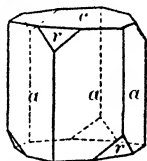
Fig. 129. Corundum.
