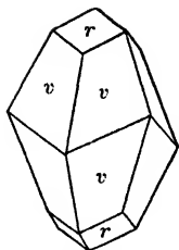
Fig. 133. Calcite.
