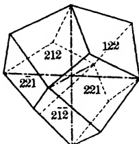
Fig. 69. Deltoïd Dodecahedron.
