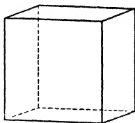
Fig. 15. Cube.
