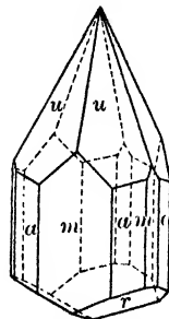
Fig. 140. Tourmaline.
