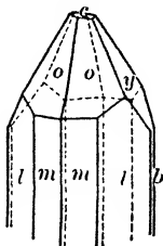
Fig. 155. Topaz
