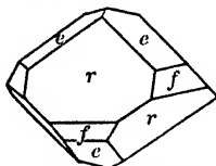
Fig. 128. Chabazite.
