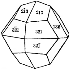
Fig. 54. Diploid.
