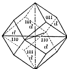
Fig. 33. Dodecahedron.
