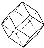
Fig. 19. Dodecahedron.
