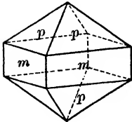
Fig. 85. Zircon.
