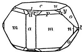
Fig. 158. Anglesite.
