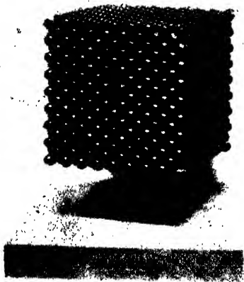
A. Cube.
