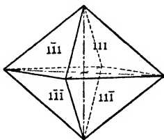
Fig. 146. Pyramid.
