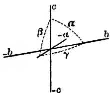
Fig. 180. Triclinic Axes.
