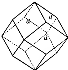
Fig. 211. Dodecahedron.
