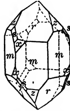
Fig. 249. Left-handed Crystal.
