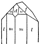
Fig. 154. Topaz.
