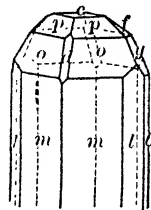
Fig. 156. Topaz.
