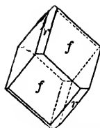
Fig. 124. Calcite.
