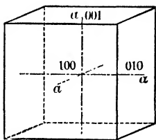
Fig. 29. Cube.
