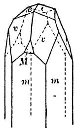
Fig. 136. Calcite.
