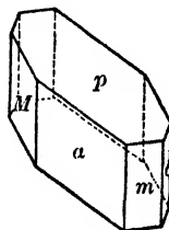
Fig. 188. Chalcantite.
