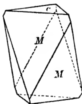
Fig. 125. Calcite.
