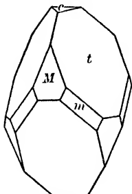
Fig. 126. Calcite.
