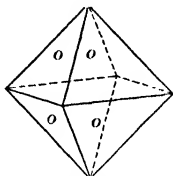
Fig. 12. Octahedron.
