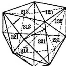
Fig. 70. Hexakistetrahedron.
