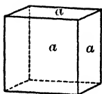
Fig. 217. Cube.
