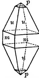
Fig. 87. Zircon.
