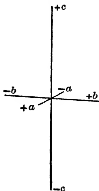
Fig. 143. Orthorhombic Axes.
