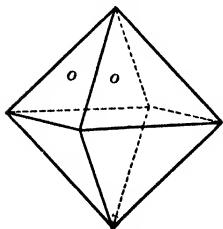
Fig. 210. Octahedron.
