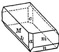
Fig. 187. Rhodonite.
