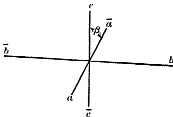
Fig. 163. Monoclinic Axes.
