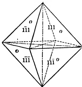
Fig. 30. Octahedron.
