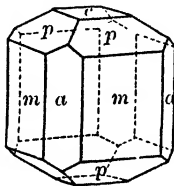
Fig. 90. Vesuvianite.
