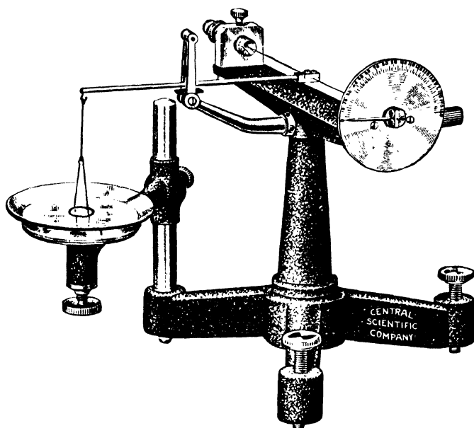
FIG. 3. du Noüy Tensiometer.†
