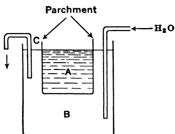
FIG. 12. Dialysis Apparatus.
