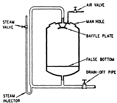
FIG. 3. Kier.
