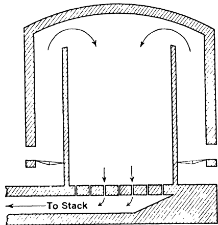
FIG. 7. Batch Kiln.
