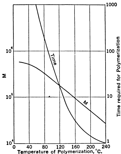
FIG. 22. Styrene Polymerization.*
