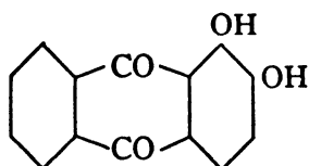
alizarine
