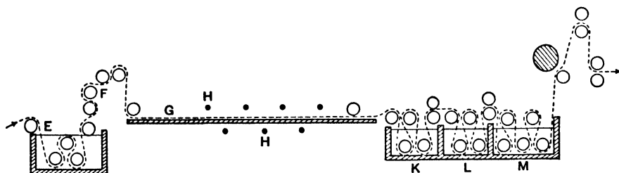
FIG. 4. Mercerizing Range.
