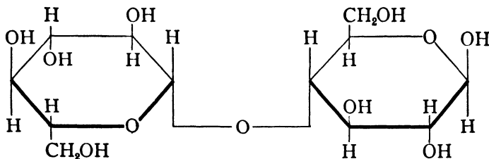
cellobiose
