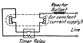
FIG. 94.—Sodium lamp circuit.
