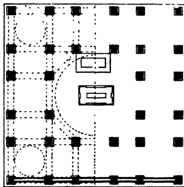
FIG. 37.—Plan of Tomb, Rânî Rupâvatî's Masjid.
