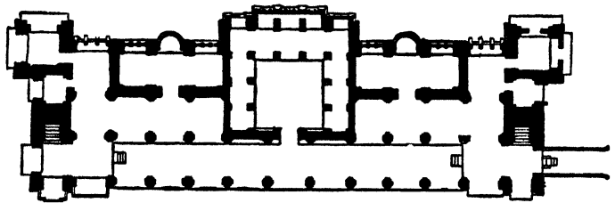
FIG. 48.—Ground Plan.
