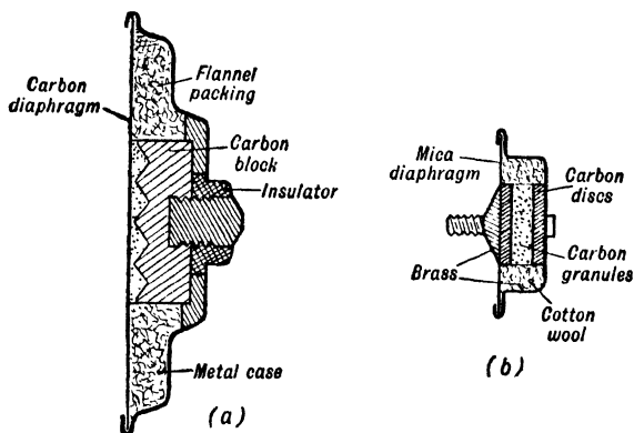
FIG. 119—Carbon Granule Microphones
