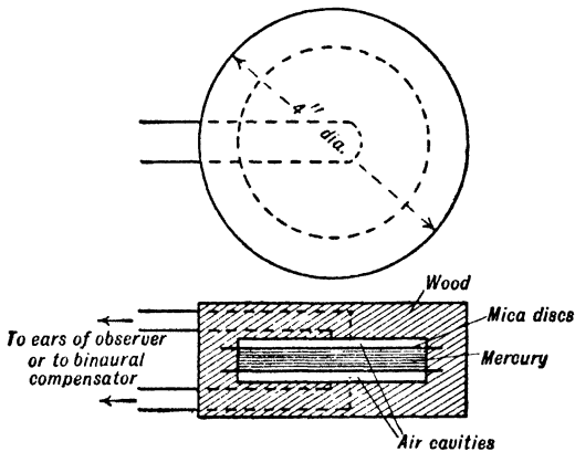
FIG. 124—Geophone
