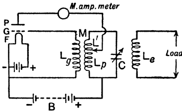
FIG. 25—Valve Oscillator
