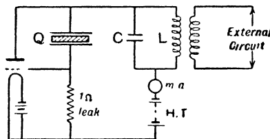
FIG. 47—Quartz Oscillator (Pierce)
