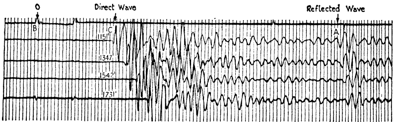
FIG. 150A—Reflection Seismograms
