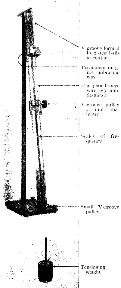
FIG. 31—Dye's 'Sonometer'
