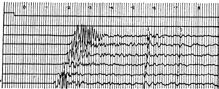
FIG. 150B—Reflection Seismograms
