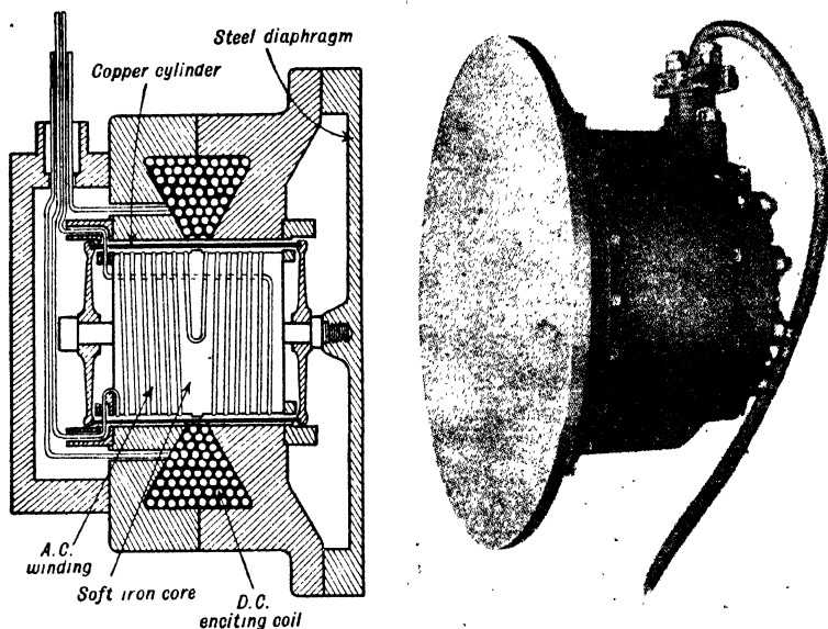
FIG. 116—Fessenden Oscillator
