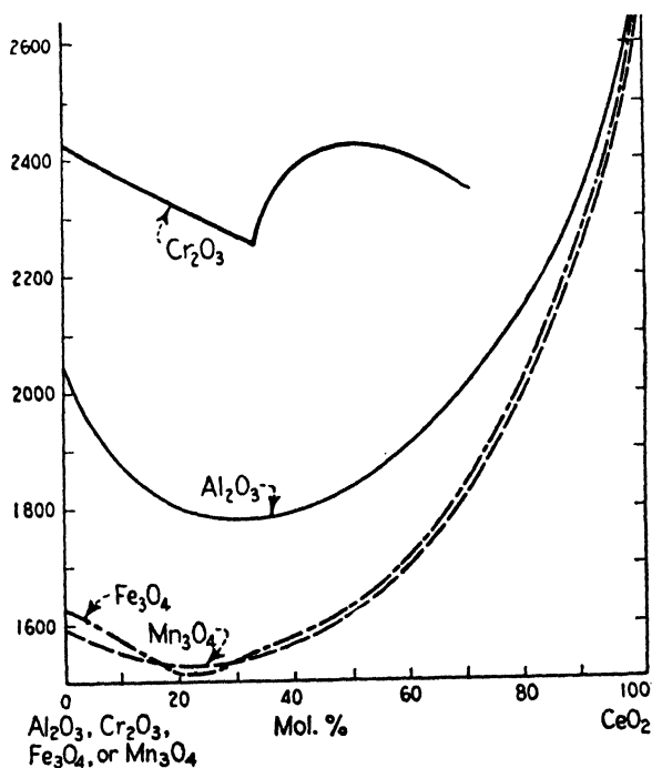
FIG. 201. Liquidus curves of systems \text{CeO}_2\text{-Al}_2\text{O}_3 , \text{CeO}_2\text{-Cr}_2\text{O}_3 , \text{CeO}_2\text{-Fe}_3\text{O}_4 , \text{CeO}_2\text{-Mn}_3\text{O}_4 . (H. von Wartenberg and K. Eckhardt, Part VIII, Z. anorg. u. allgem. Chem. , 232 , 184, 1937.)
