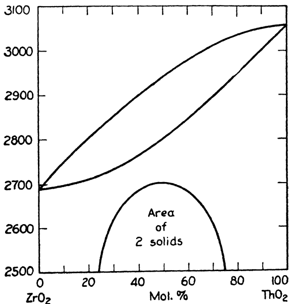
FIG. 217. System ThO 2 -ZrO 2 ; probable diagram. (O. Ruff, F. Ebert, and H. Wöitinek, Z. anorg. u. allgem. Chem. , 180 , 255, 1929.)
