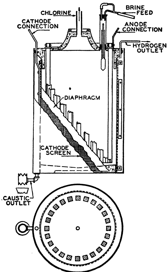
FIG. 44.—Gibbs-Vorce cell.
