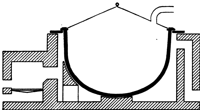
FIG. 49.—Caustic pot.
