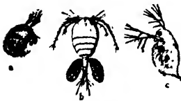
FIG. 24.—Crustacea: a, Cypris ; b, Cyclops ; c, Daphnia .
