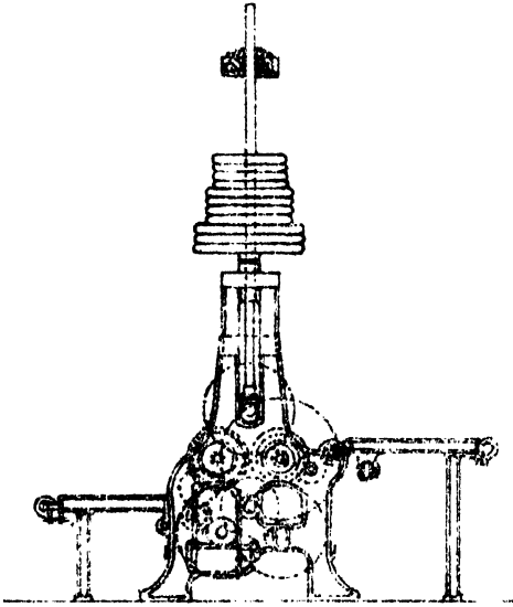
END ELEVATION
