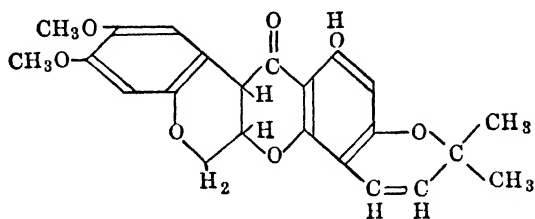
Toxicarol
