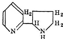
\alpha - nornicotine
