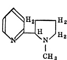
\alpha -nicotine
