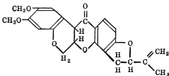
Rotenone
