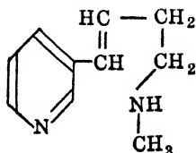
Metanicotine
