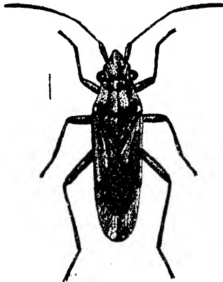
Fig. 83.-- Nysiodes typus .
