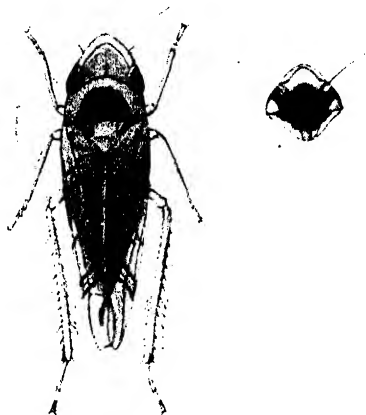
Fig. 54.— Bolanusoides heros .
