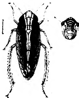
Fig. 35.— Hussa i
