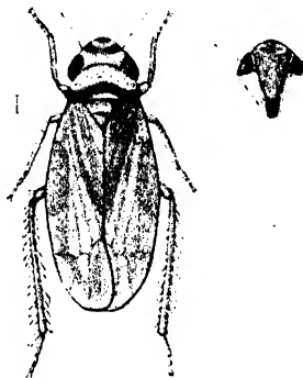
Fig. 55.— Empoascanara prima .
