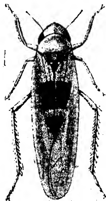
Fig. 61.— Typhlocyba? incerta .
