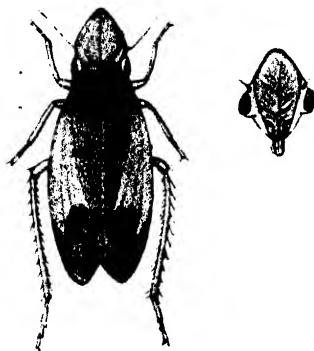
Fig. 15.— Ophiuchus princeps .
