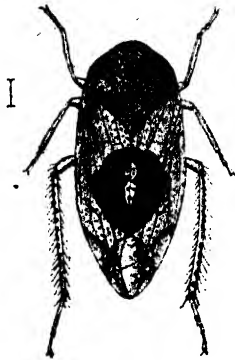
Fig. 32.— Eutettix bengalensis .
