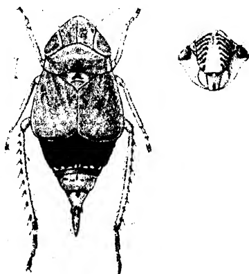
Fig. 50.— Leofa mysorensis .
