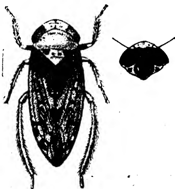
Fig. 21.— Carvaka picturata .
