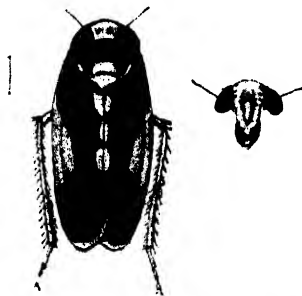
Fig. 25.— Æternus hieroglyphicus .
