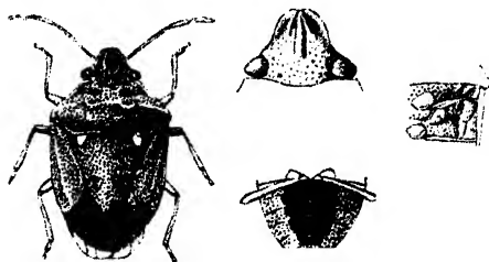
Fig. 68.— Neocarbula capitata .
