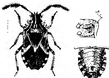
Fig. 67.— Phricodus hystrix .
