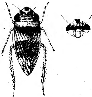
Fig. 48.— Postumus facialis .
