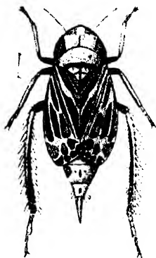
Fig. 27.— Prasutagus pulcheilus .
