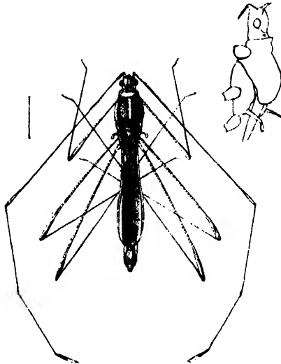
Fig. 80.— Taprobanus gravelyi .
