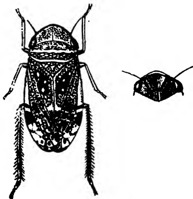
Fig. 11.— Vulturinus ornatus .
