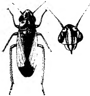
Fig. 2.— Omaranus typicus .
