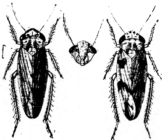
Fig. 31.— Divitiacus primus .
