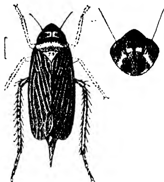
Fig. 26.— Trebellius albifrons .
