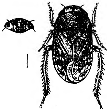
Fig. 7.— Penthimia mudonensis .
