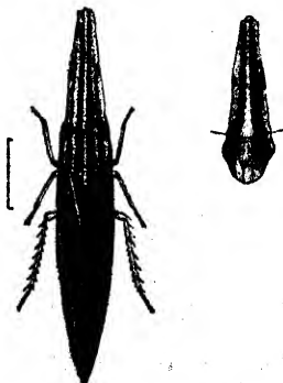
Fig. 14.— Bumizana elongata .
