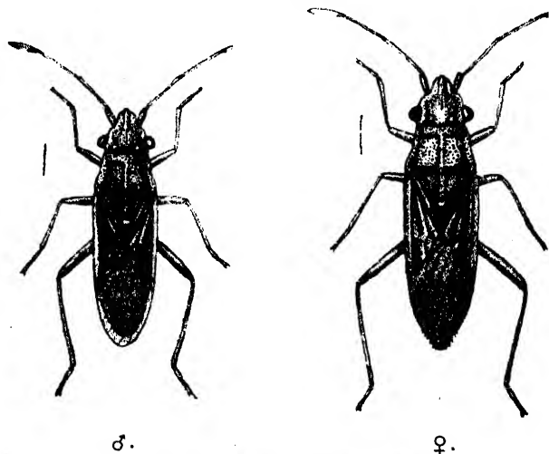
Fig. 79.— Agraphopus lethierryi .
