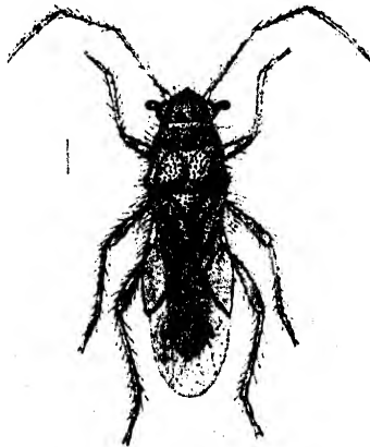
Fig. 85.— Ossipaga ceylanica .
