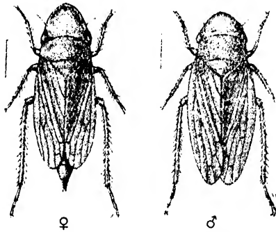
Fig. 13.— Parabolocratius rusticus .
