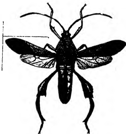
Fig. 75.— Xyrophoreus tonsor .
