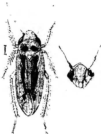
Fig. 44.— Crispina nigristigma .
