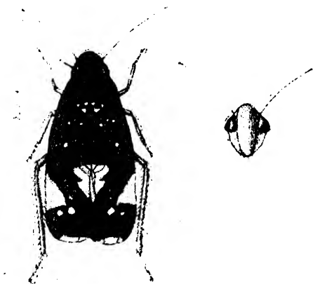
Fig. 59.— Augulus typicus .
