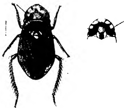
Fig. 10.— Malichus capitatus .
