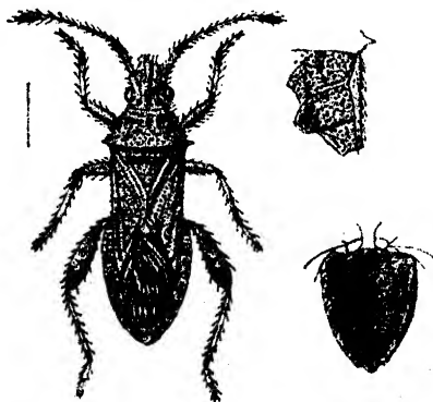
Fig. 76.— Neohoplotomia typica .
