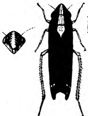
Fig. 4.— Faenius lynchi .
