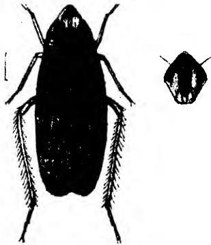
Fig. 23.— Coroticus tessellatus .
