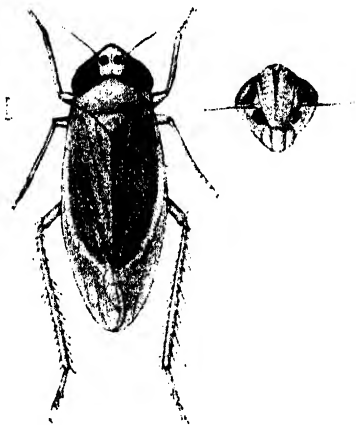
Fig. 56.— Paivanana indra .
