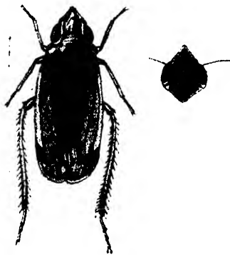
Fig. 24.— Cunedita phæops .
