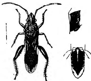
Fig. 77.— Daclera levana .
