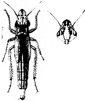
Fig. 18.— Didius sexualis .
