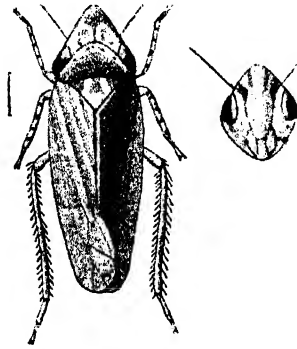
Fig. 41.— Zizyphoides indicus .
