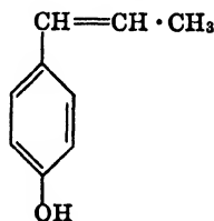
p -Anol
