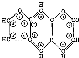
Psoralene (linear type)
