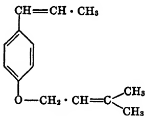
Feniculin
