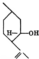
d - \alpha -isopulegol
