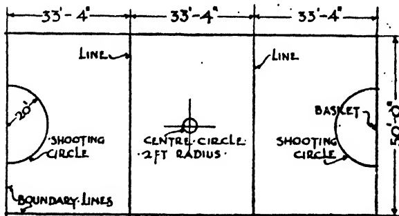
BASKET-BALL COURT FOR MATCHES
