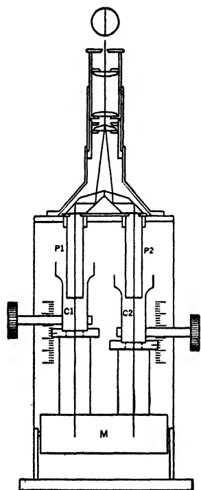
FIG. 29. Duboscq Colorimeter.
