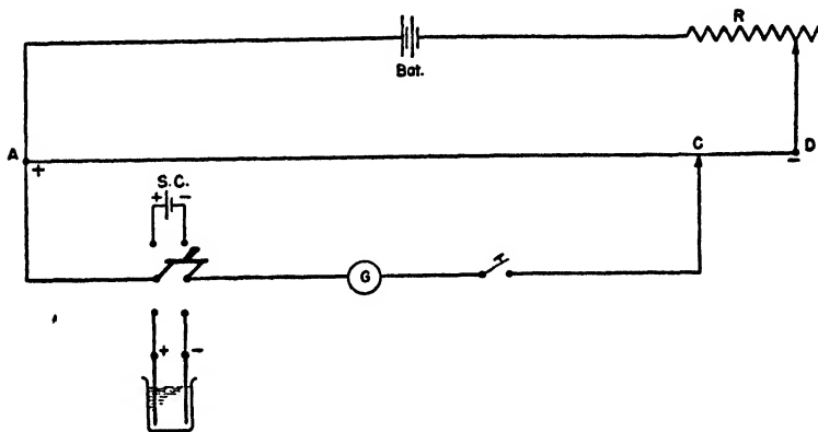
FIG. 21. Potentiometer.
