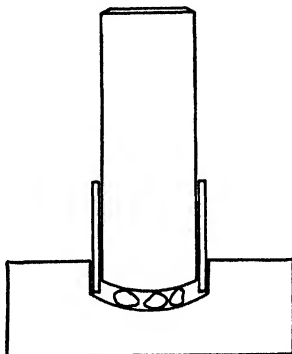
FIG. 8. Diamond Mortar.
