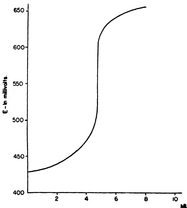
FIG. 24. Titration Curve.
