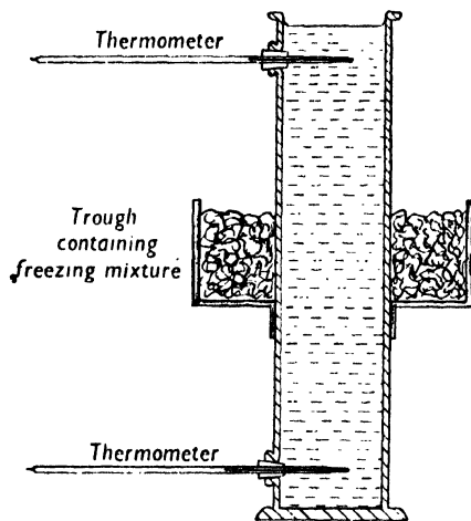
FIG. 43. HOPE'S APPARATUS
