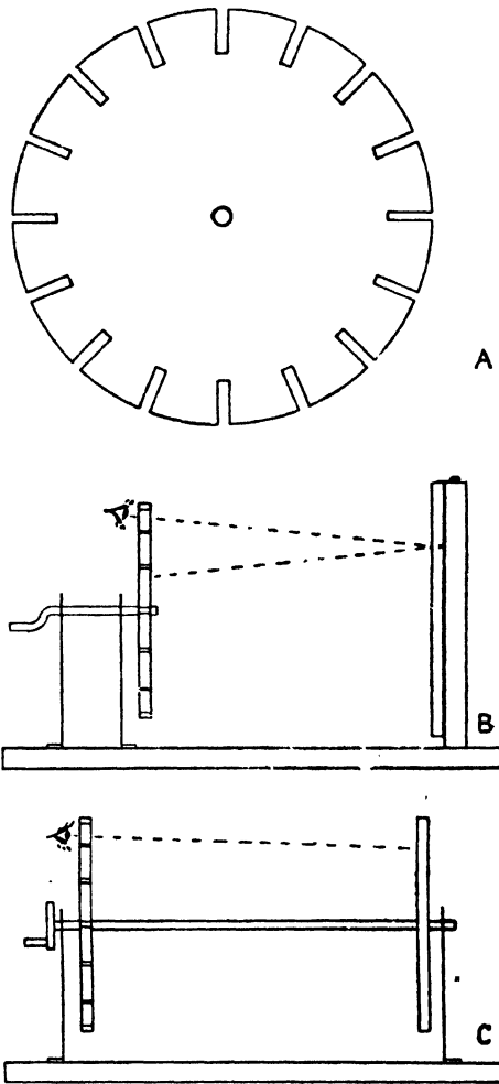
FIG. 57. THE DISC APPARATUS
