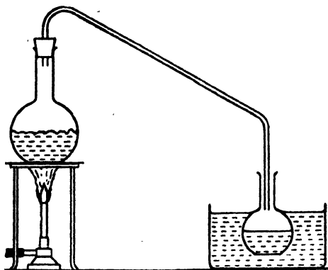
FIG. 48. DISTILLATION APPARATUS
