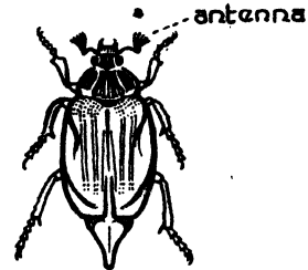
FIG. 4. COCKCHAFER
