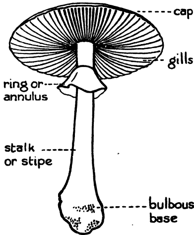
FIG. 12. TOADSTOOL
