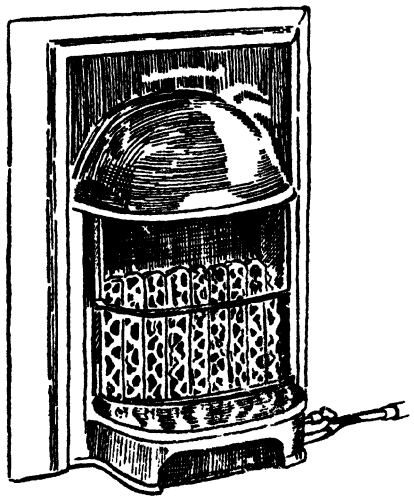
FIG. 27. GAS FIRE
