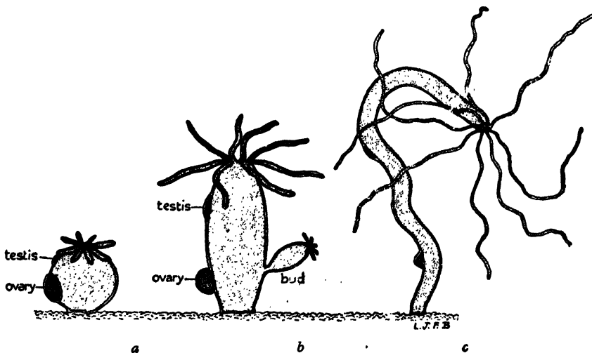
FIG. 44. HYDRA
