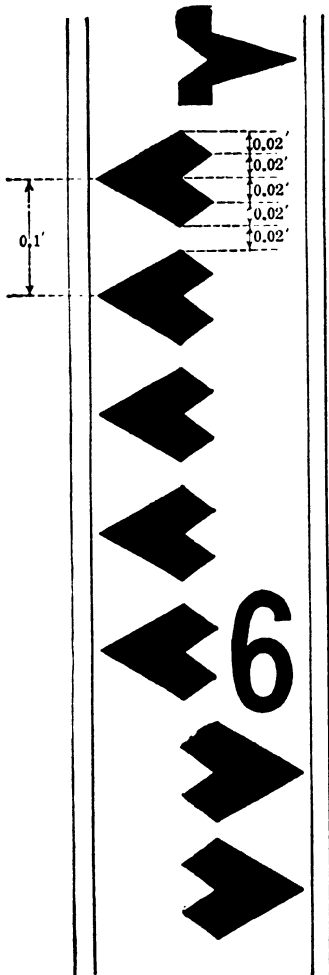
FIG. 305.—Stadia rod.
