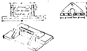
FIG. 342.—Split float.
