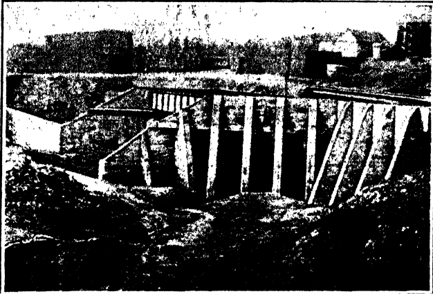
FIG. 121.—Counterfort abutment, K. C. M. & O. R. R.
