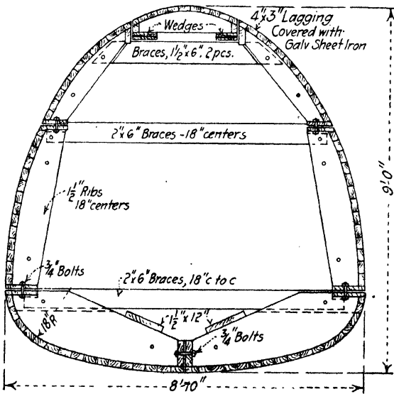
FIG. 205.—Collapsible center for a conduit.
