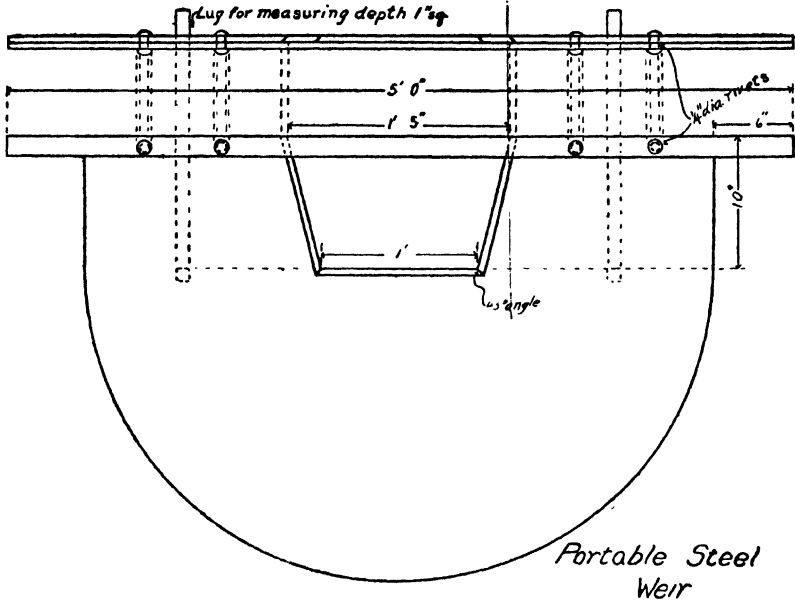
Fig. 21: — Portable steel weir. (Utah Agr. Exp. Sta. Circular 36.)
