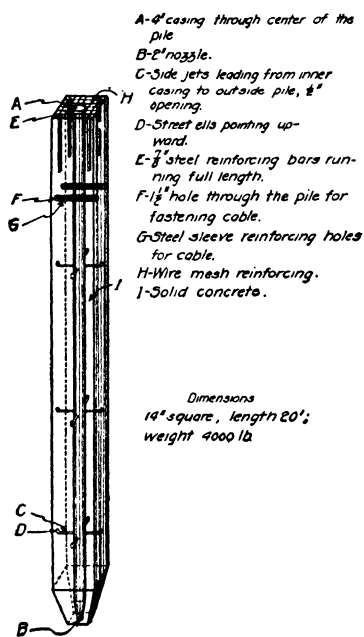
FIG. 33.—Bignell pile.
