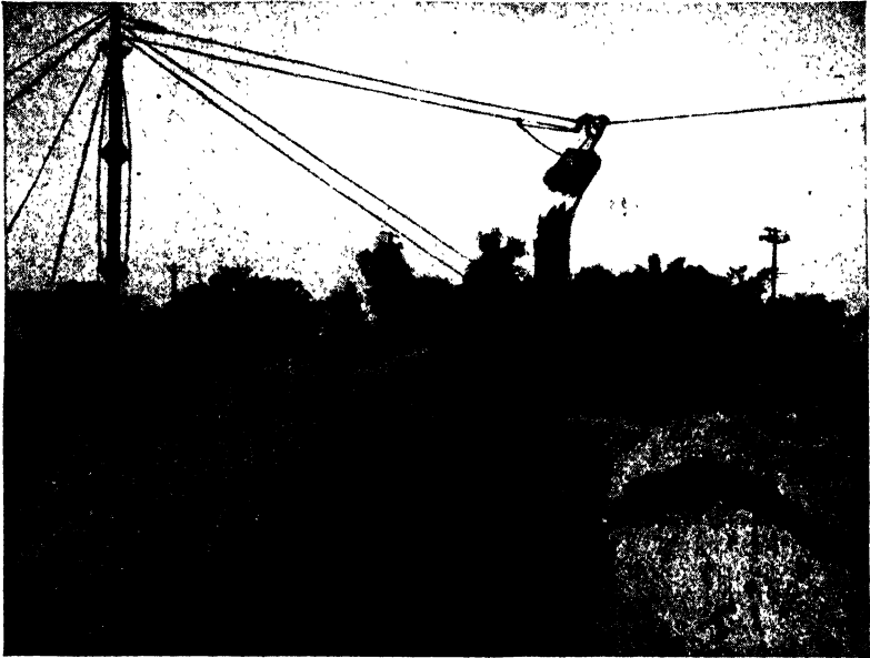
FIG. 15a.—Slack-line cableway excavator. (Courtesy of Sauerman Bros.)
