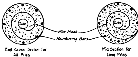
FIG. 32.—Chenoweth pile.
