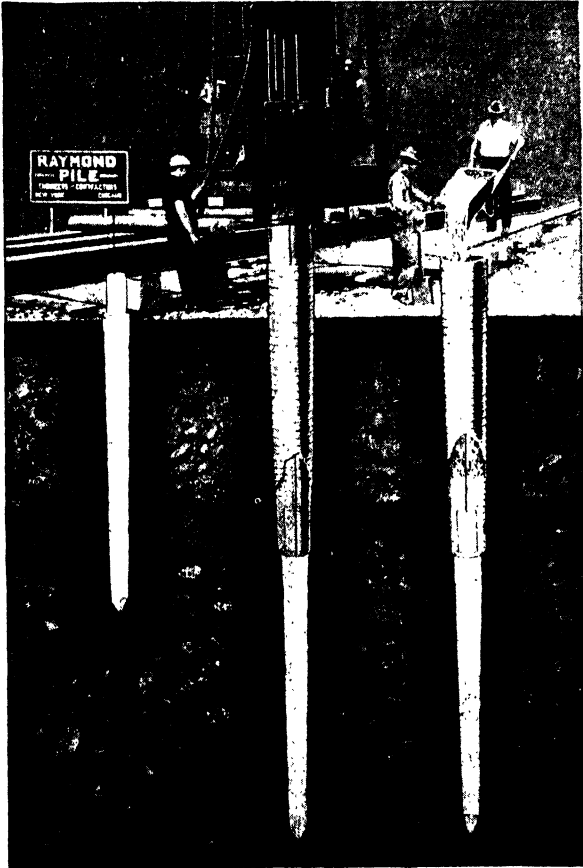
FIG. 48.—Placing Raymond composite pile.
