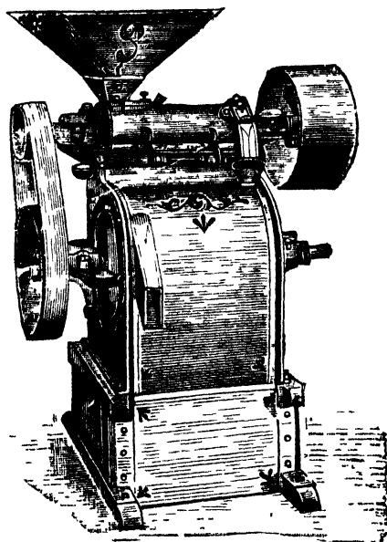
FIG. 62.—ENGELBERG HULLER.
