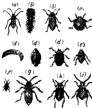
FIG. 108.—COLEOPTERA.
