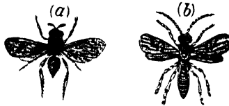
FIG. 107.—HYMENOPTERA.
