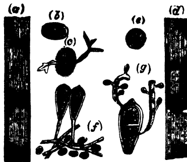
FIG. 117.—PUCCINIA GRAMINIS.
