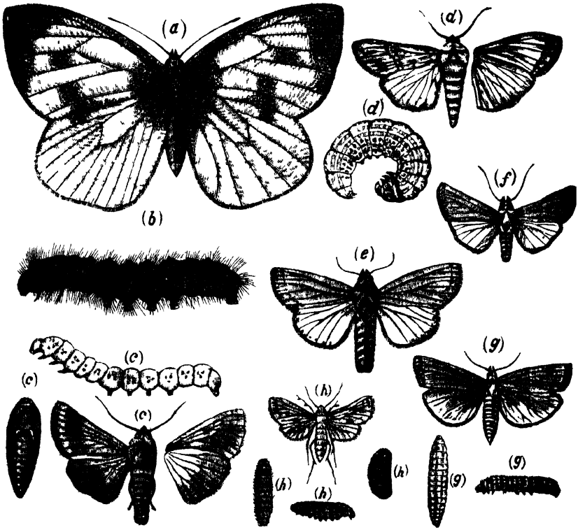
FIG 109.—LEPIDOPTERA.
