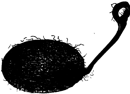
FIG. 80.—BUGUI COCOON.
