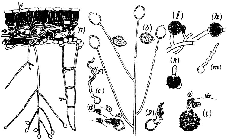
FIG. 116.—PHYTOPHTHORA INFESTANS.
