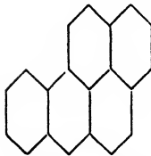
1, 2-Benzopyrene
