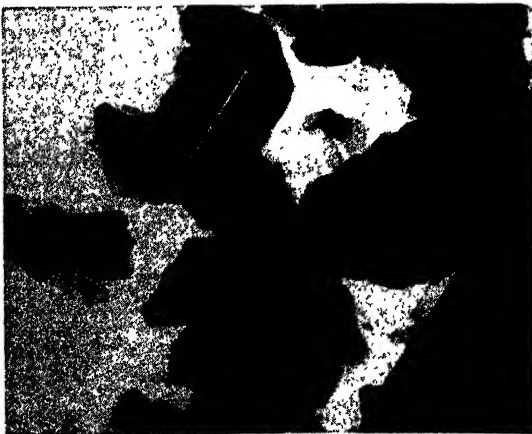
FIGURE 19a. Kaolinite.
