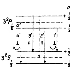
Fig. 25. Magnetic sublevels for the Na-line D_1 .
