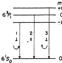
Fig. 24. Magnetic sublevels for the Hg-line 2537A.
